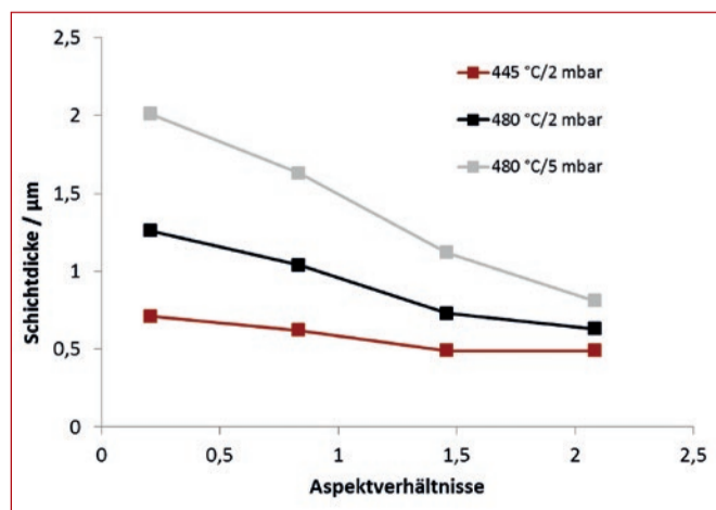
Abbildung 4: Für den modifizierten Formeinsatz der Firma Werner Bauser GmbH ergeben sich ebenfalls bei geringeren Temperaturen gleichmäßigere Schichtdickenverteilungen.
