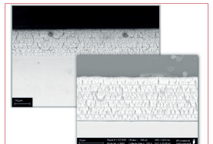
Abbildung 5: Rasterelektronenmikroskop-Aufnahme eines Querschnitts einer beschichteten Stahlprobe mit einer Kombinationsschicht, bestehend aus kristallinem und amorphem Zirkoniumdioxid.
