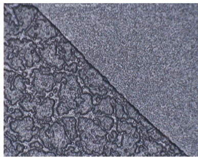
Unterschied einer glatten Keramik-Oberfläche zu einer laserstrukturierten rauhen Oberfläche
