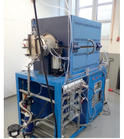
Abbildung 2 (r.): Der CVD-Reaktor der gemeinnützigen KIMW Forschungs-GmbH.
