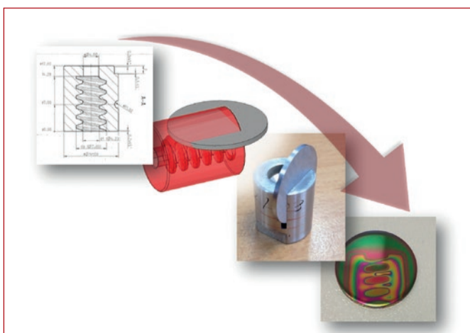
Abbildung 3: Es wurden Formeinsätze modifiziert, um sie mit flächigen Probekörpern versehen und nach der Beschichtung zur Messung der Schichtdicke innerhalb der Kavität heranziehen zu können.
