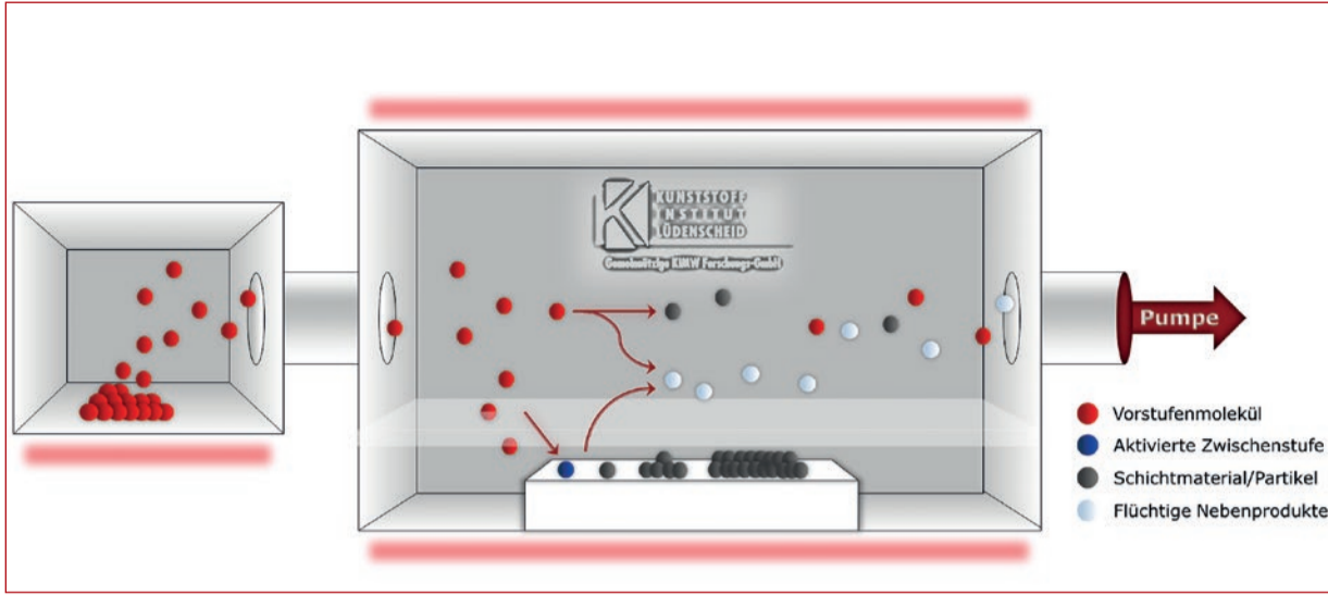
Abbildung 1 (l.): Schematischer Aufbau eines CVD-Reaktors, in dem es zur thermisch induzierten Zersetzung der Vorstufenmoleküle sowie zur Bildung des Schichtmaterials auf der Substratoberfläche kommt.
